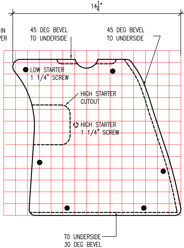
TOEBOARD-FRONT-R.H.
