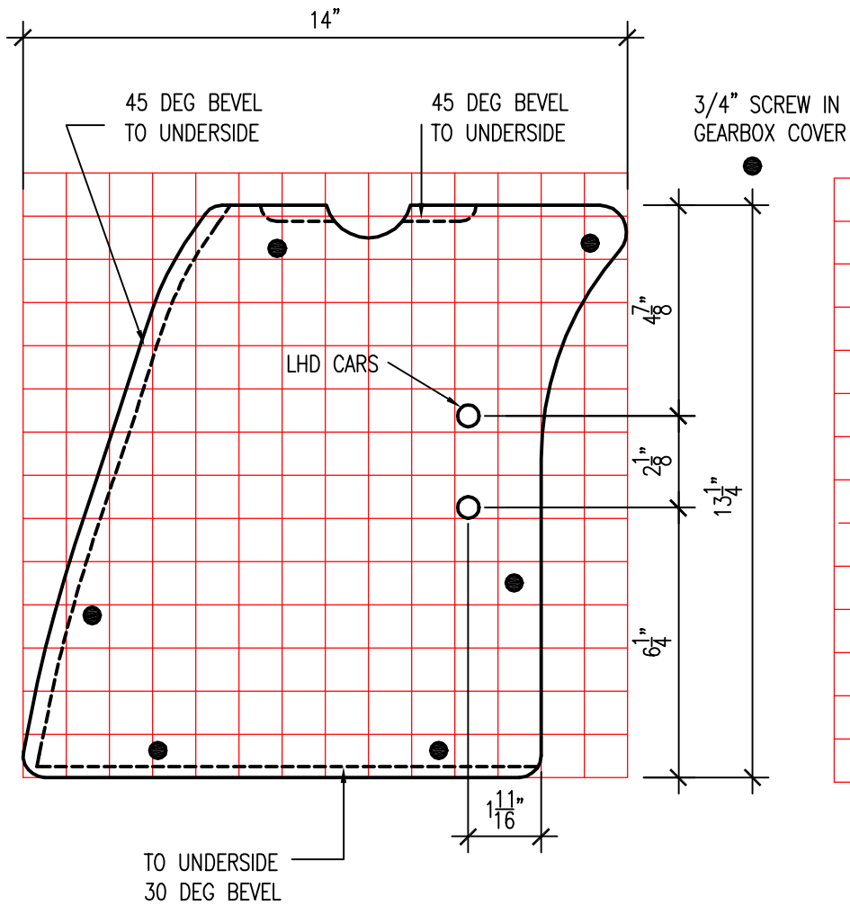
TOEBOARD-FRONT-L.H.
